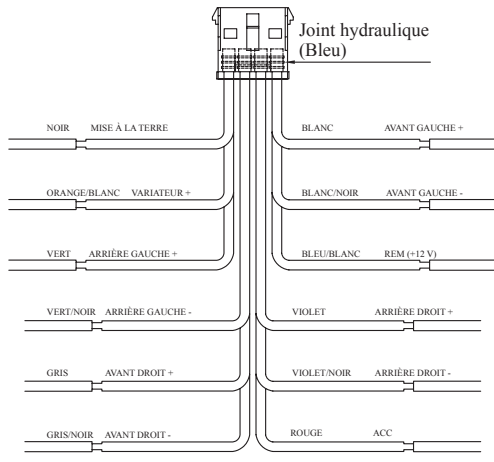
FAISCEAU 12 BROCHES
