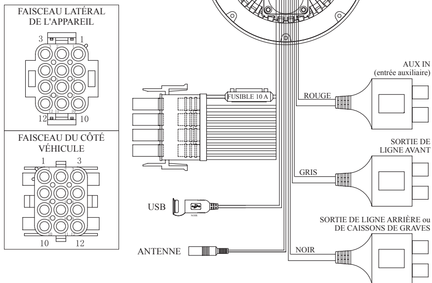
FAISCEAU 12 BROCHES
