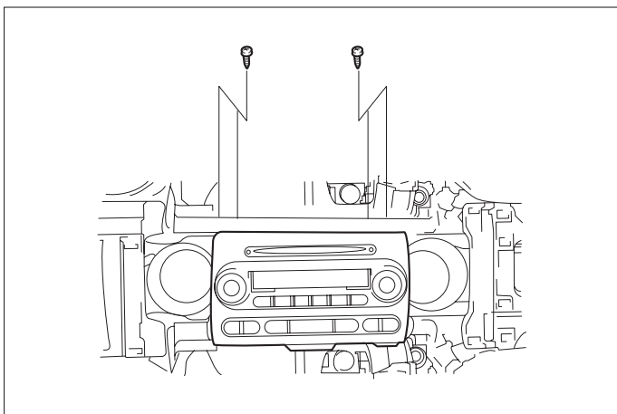
(5) 固定用ビス(4本)を外し、オーディオA' ssyを取外します。
