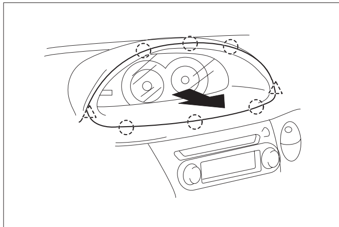
(2) メーターフードを取外します。
