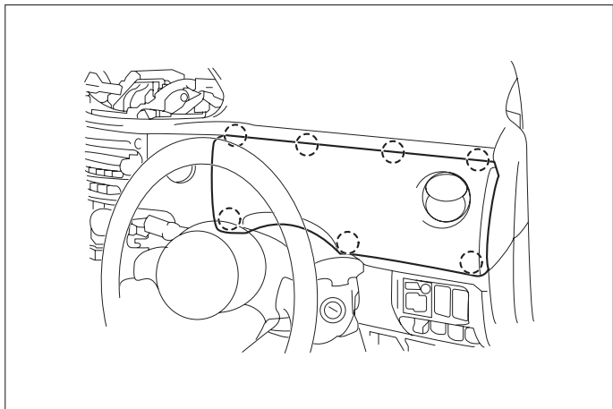
(1) インstrumentパネル(RH)を取外します。
