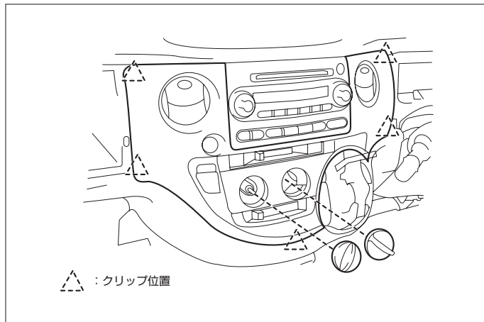
(4) ヒーターコントロールノブ(2ヶ)を取外し、パネル固定用ビス(2本)を取外し、instrumentセンターパネルを取外します。
