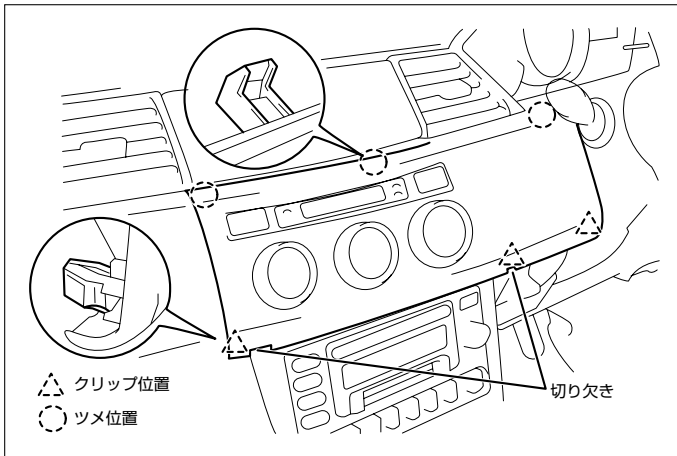
(1) センタークラスターモジュールコントロールA'ssyを取外します。
