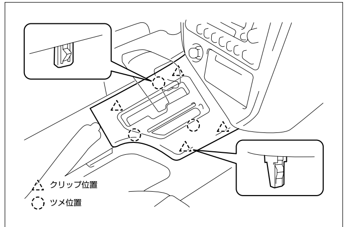
(2) コントロールパネルアッパーを取外します。
