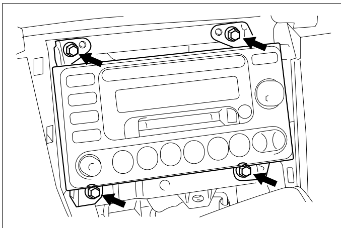
(5) オーディオA'ssyを取外します。
