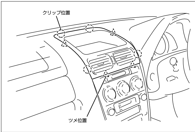
(1) インストルメントクラスタフィニッシュパネルを取外します。 (除くマルチディスプレイ装着車)
