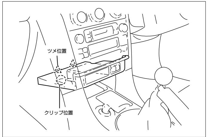
(2) インストルメントクラスタフィニッシュパネルロアを取外します。 (オーディオ装着車)
