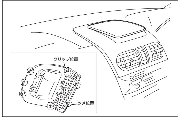
(2) クラスタリッドCを取外します。
