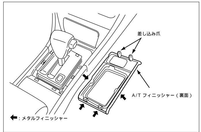
(2)A / Tシフトカバーを取外します。
