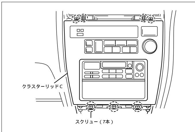
(3)センタークラスターC A ssyを取外します。
