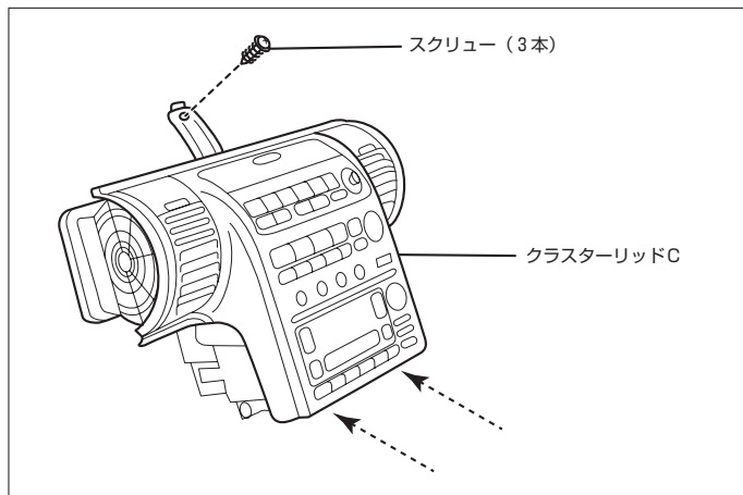
(6) クラスタリッドC A'ssyを取外します。
