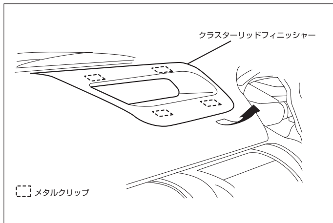
(4) クラスタリッドフィニッシャーを取外します。
