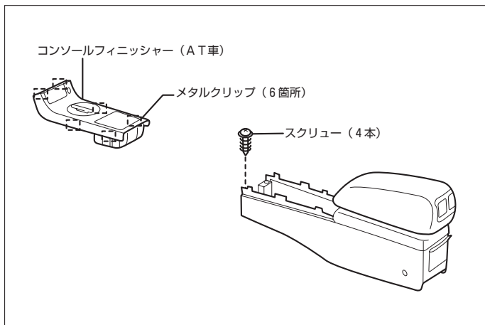
(3) コンソールフィニッシャーカバー(AT)を取外します。
