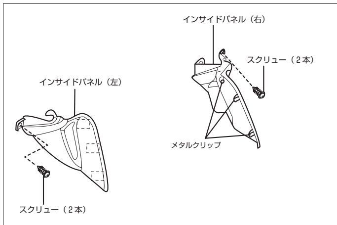
(5) インサイドパネル(左右)を取外します。
