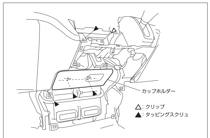
(4) カップホルダーを取外します。
