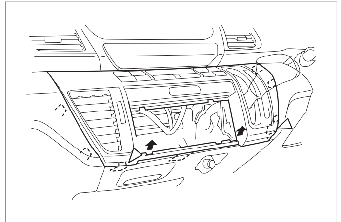
(2) センターポケットを外し、インストルメントセンターミドルパネルを取外します。
