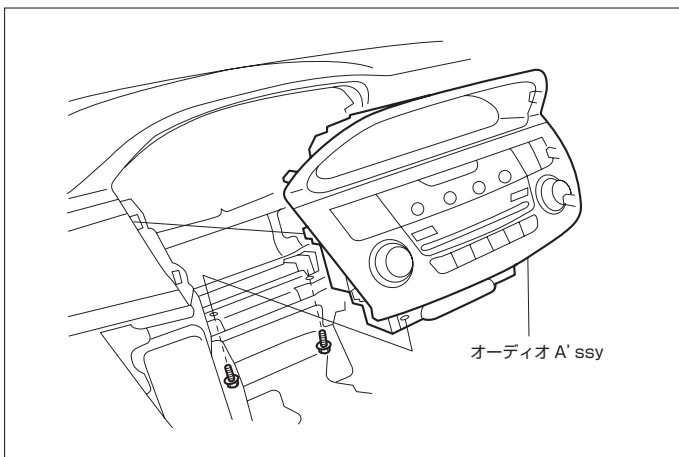
(5) オーディオA'ssyを取外します。
