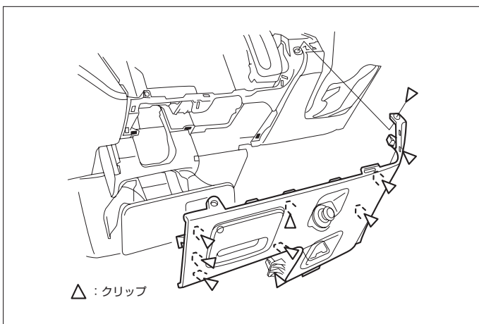
(3) カップホルダーを引き出し、センターロアパネルを取外します。
