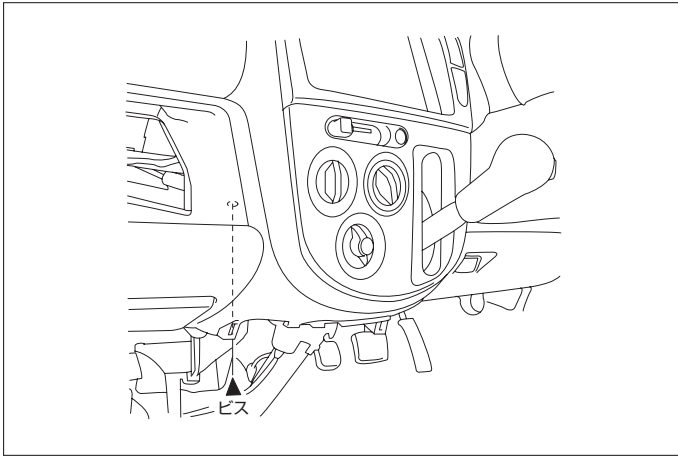
(3) 固定用ボトルを取外し、ヒーターコントロールユニットを取外します。(マニュアルA/C場合は、ケーブルを外す必要があります)
