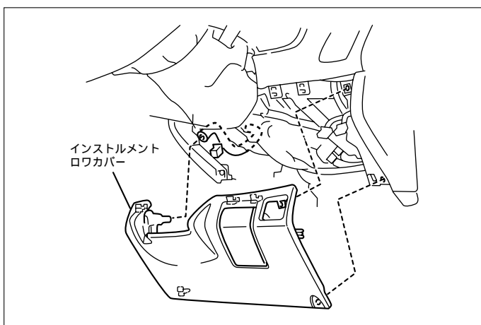
(3)インストルメントロウパネルを取外します。
