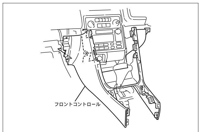
(4)グローブボックスを下げ、フロントコンソールを取外します。 (5)オーディオA ssyを取外します。
