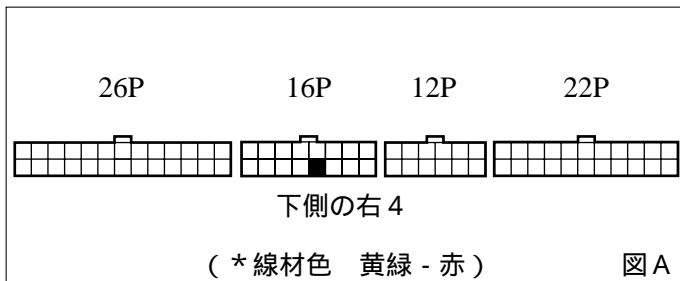
車速信号用コネクタ接続位置と線材色 G20A PGM-FI , G25A PGM-FI
