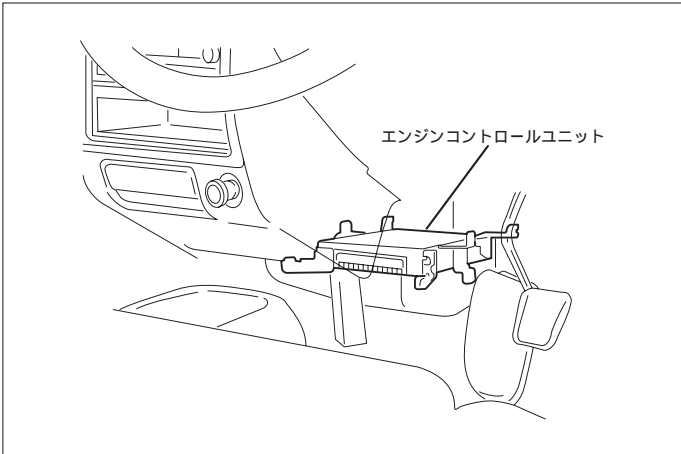
(1) センターパネルの奥側にエンジンコントロールユニットが取り付けられています。
