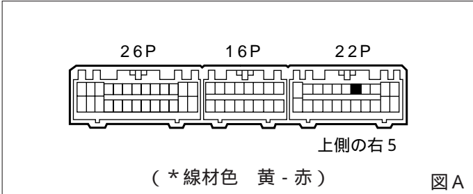
車速信号用コネクター接続位置と線材色 HE-EG , HE-EP
