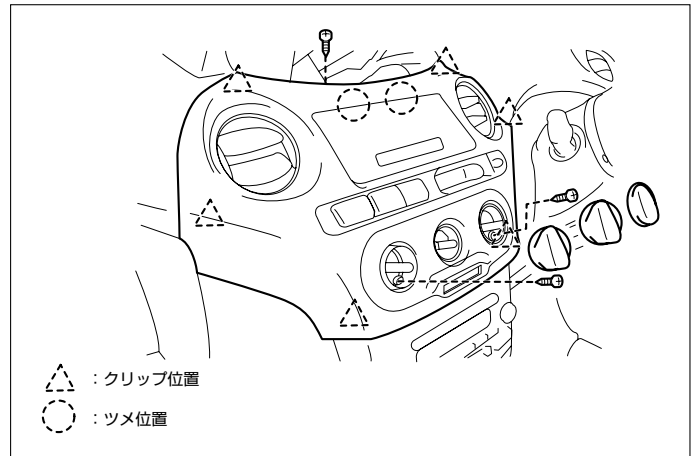
(2) インストルメントクラスターフィニッシュパネルを取外します。 (コネクター類を外します)
