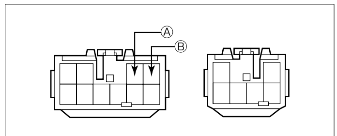
Ⓐ：ACC電源⊕ (*線材色 灰) Ⓑ：バックアップ電源⊕ (*線材色 青-黄)
