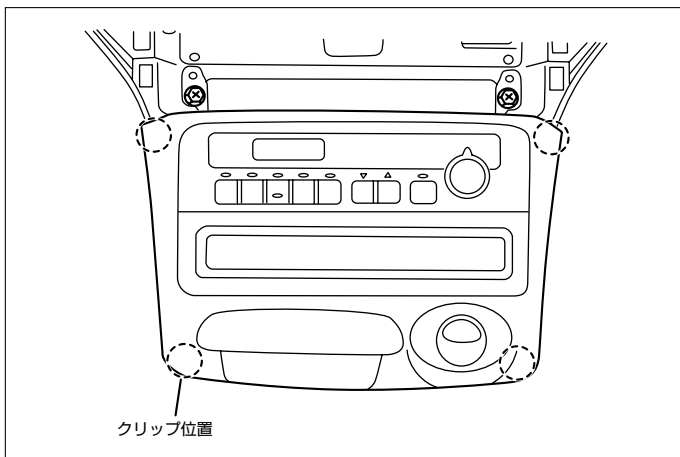
(3) インストルメントクラスターフィニッシュパネルローアを取外します。
