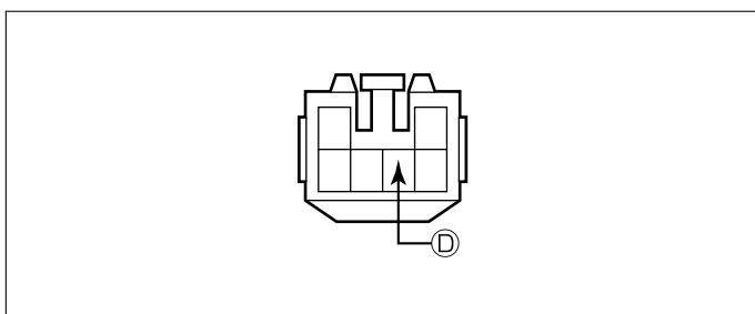
Ⓓ：バックランプ電源⊕ (*線材色 赤-白)
